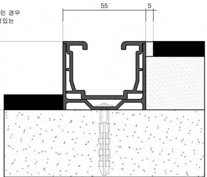
○ 매립형 하부레일을 단차 매립형으로 사용하는 경우 SC : none
