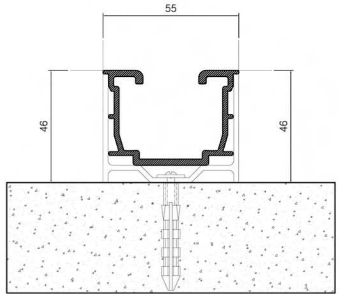
○ 매립형 하부 구조레일 설치하기 SC : none
