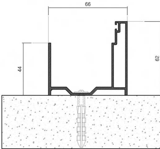
노출형 하부가틀 설치하기 SC : none
