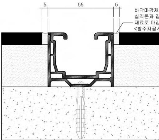
○ 매립형 하부레일 조립결과 SC : none
