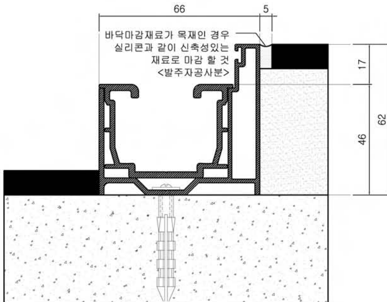
노출형 하부레일을 단차 매립형으로 사용하는 경우 - 2 SC : none
