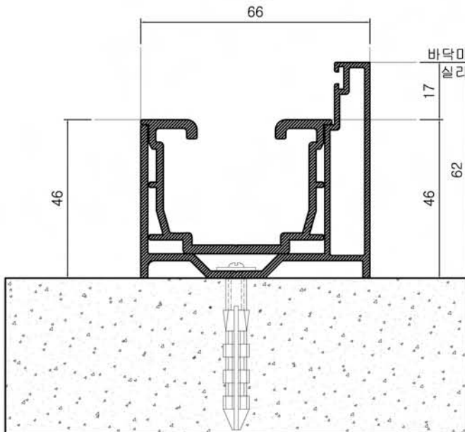
노출형 하부레일 조립결과 SC : none
