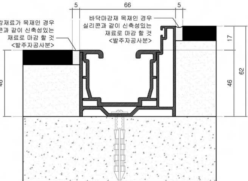
노출형 하부레일을 단차 매립형으로 사용하는 경우 - 1 SC : none
